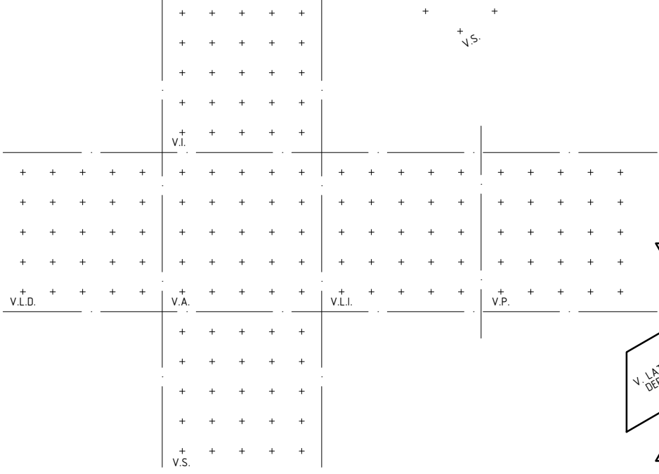
ISO-E SISTEMA DE PROYECCIÓN EUROPEO (PRIMER CUADRANTE)
