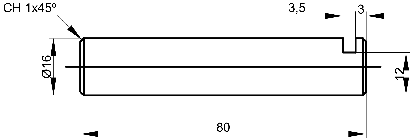
EJE
