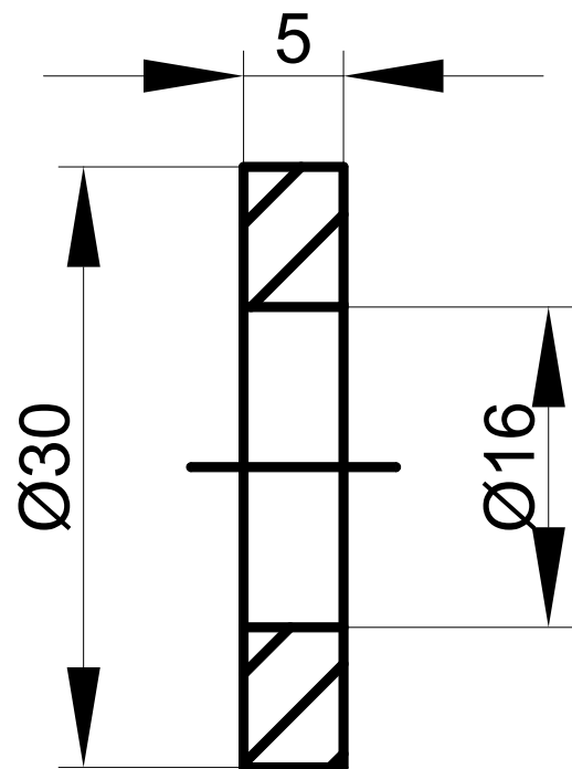
ARANDELA
