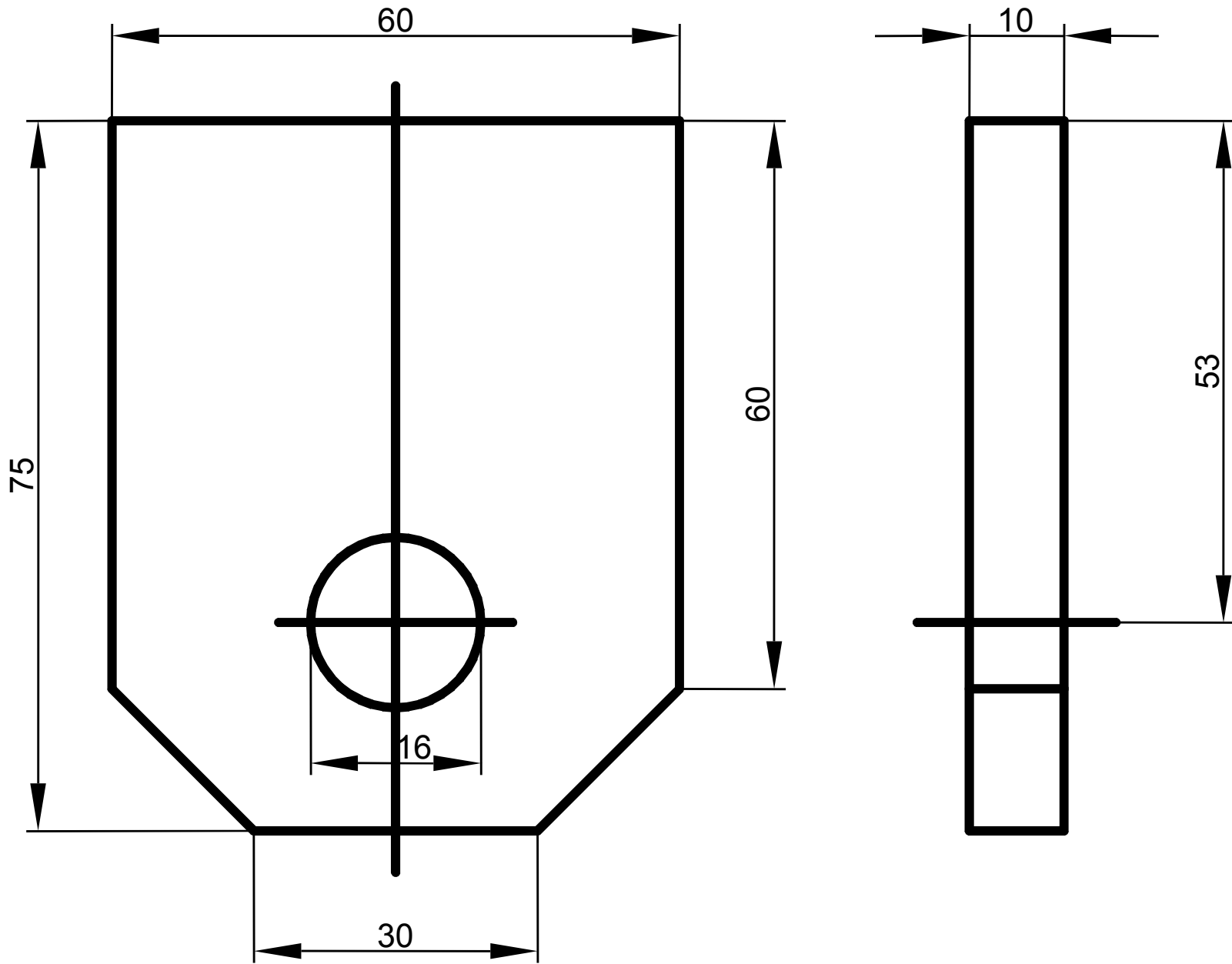
SOPORTE DERECHO
