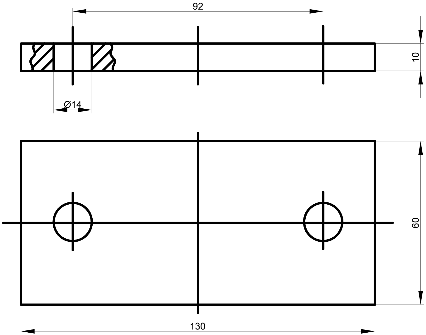
PLACA BASE
