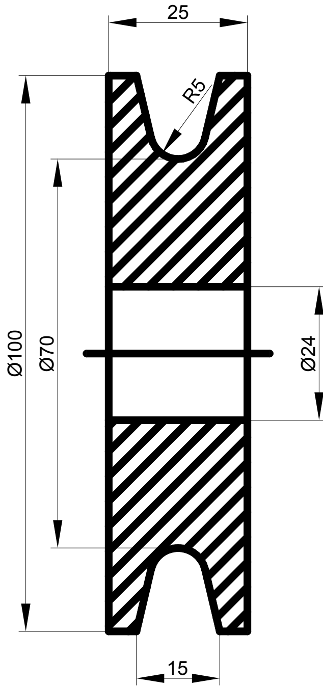
POLEA
